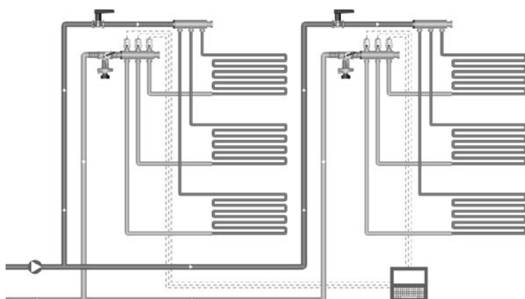
Балансировка перед коллектором системы внутрипольного отопления (Heizen Auto+ Heizen Lock)
